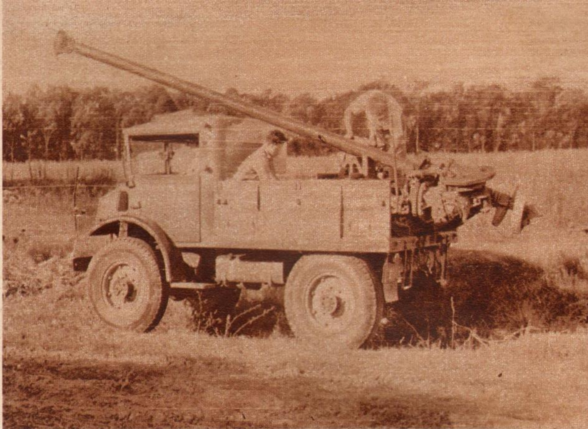
Llegan a 53 las Brigadas Móviles con que cuenta Teléfonos del Estado. Cada una de ellas está compuesta por doce hombres, perfectamente equipados con herramientas de calidad y elementos mecánicos de auxilio, como camiones perforadores de hoyos y colocadores de postes.
