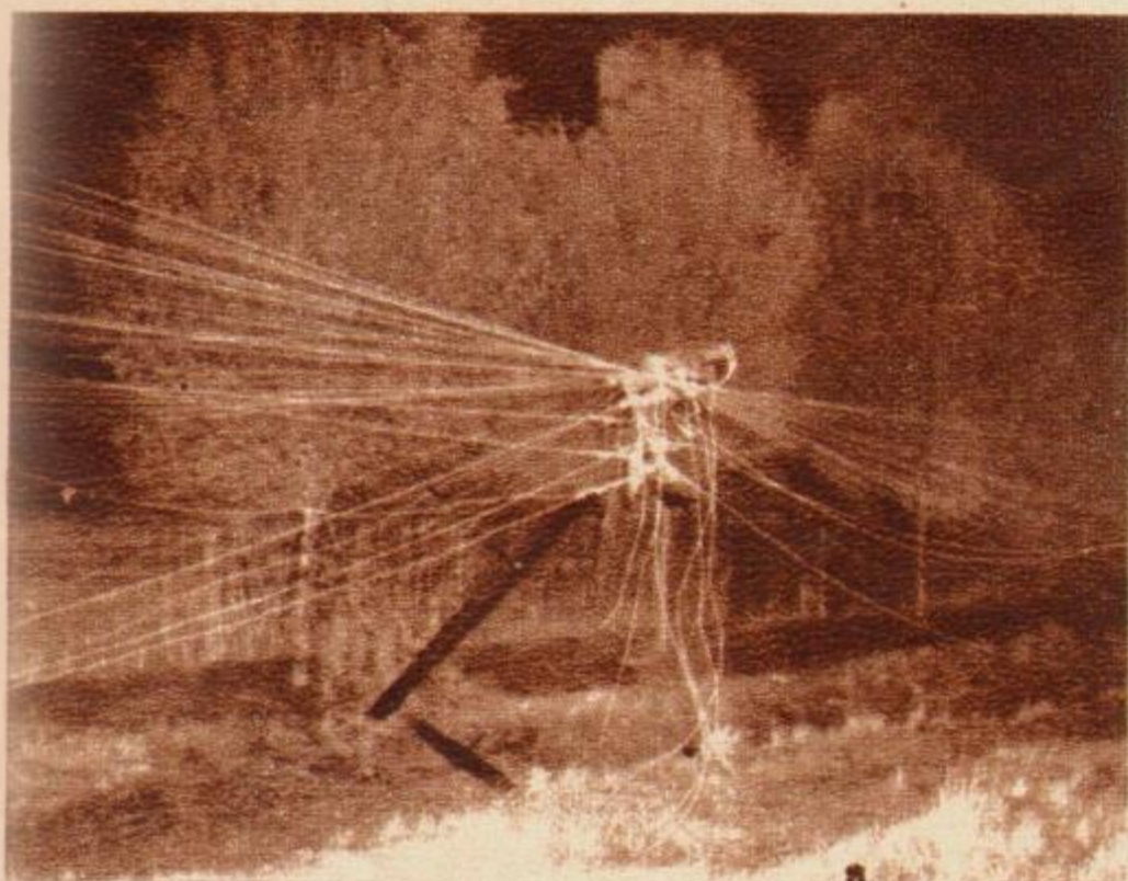
La foto muestra el estado en que quedó uno de los postes de la línea Capital Federal - Mar del Plata, a la altura de Glew, después de la tormenta. Las Brigadas Móviles repararon el daño en sólo cuatro horas.
