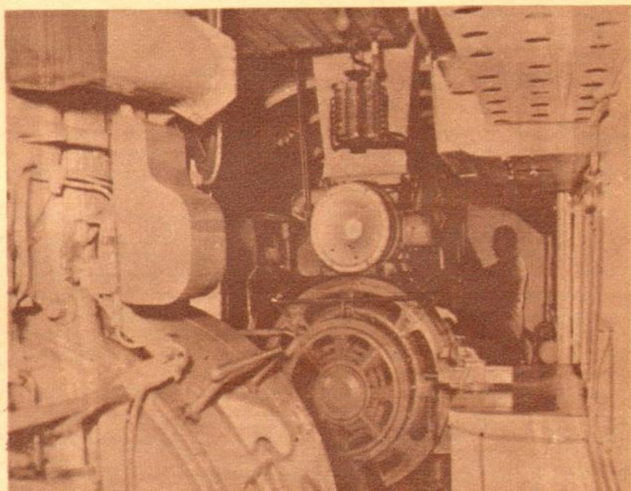
Perspectivas de dos de los cuatro motores diésel que producen la energía eléctrica de la "Argentina". Nótese la amplitud de los espacios para el movimiento de los mecánicos y electricistas.
