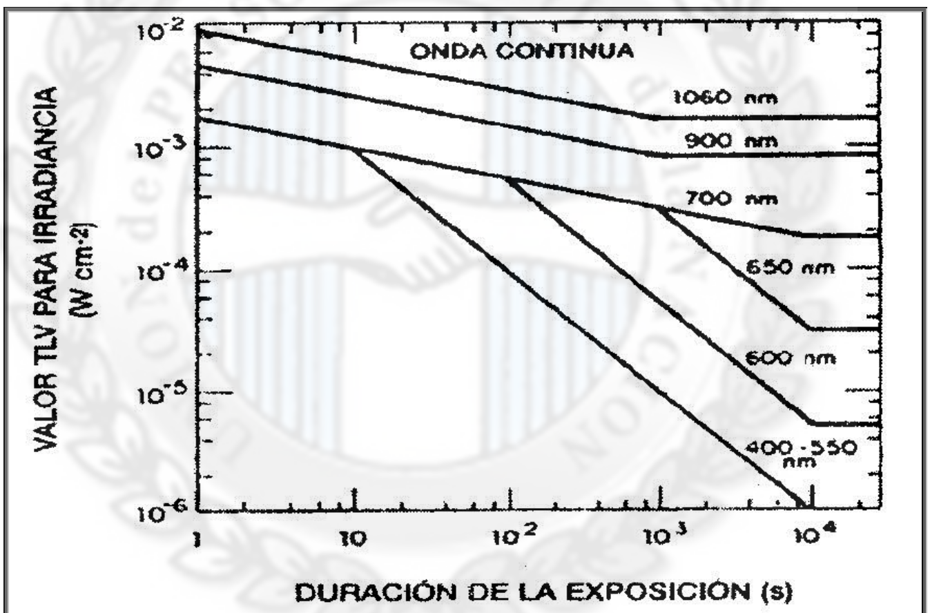
Figura 2b. Valor TLV para la exposición ocular directa del rayo láser de onda continua (400-1400 nm).
