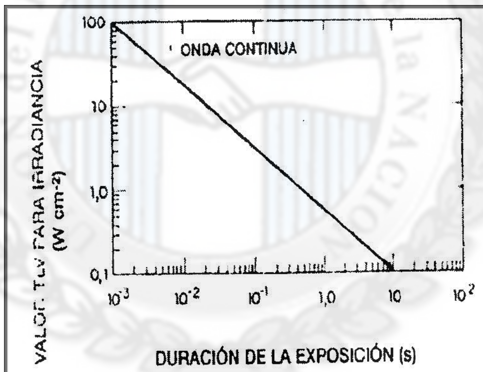
Figura 3b. Valor TLV para exposición de la piel y los ojos a láser de onda continua para radiación infrarroja lejana.
