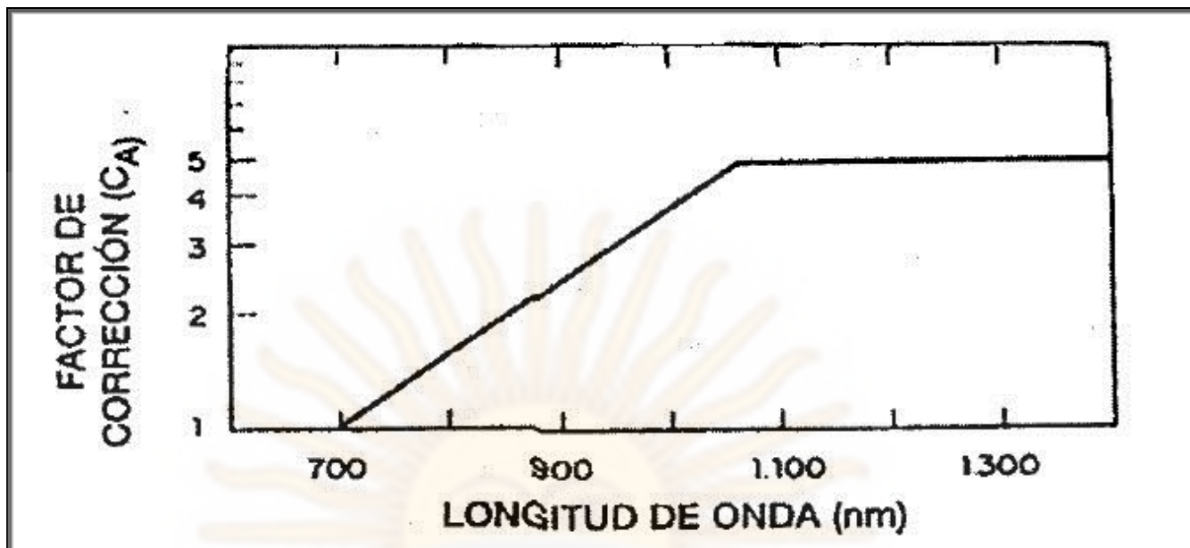
Figura 1. Factor de corrección de los valores TLV para \lambda = 700-1400\text{nm}^*
