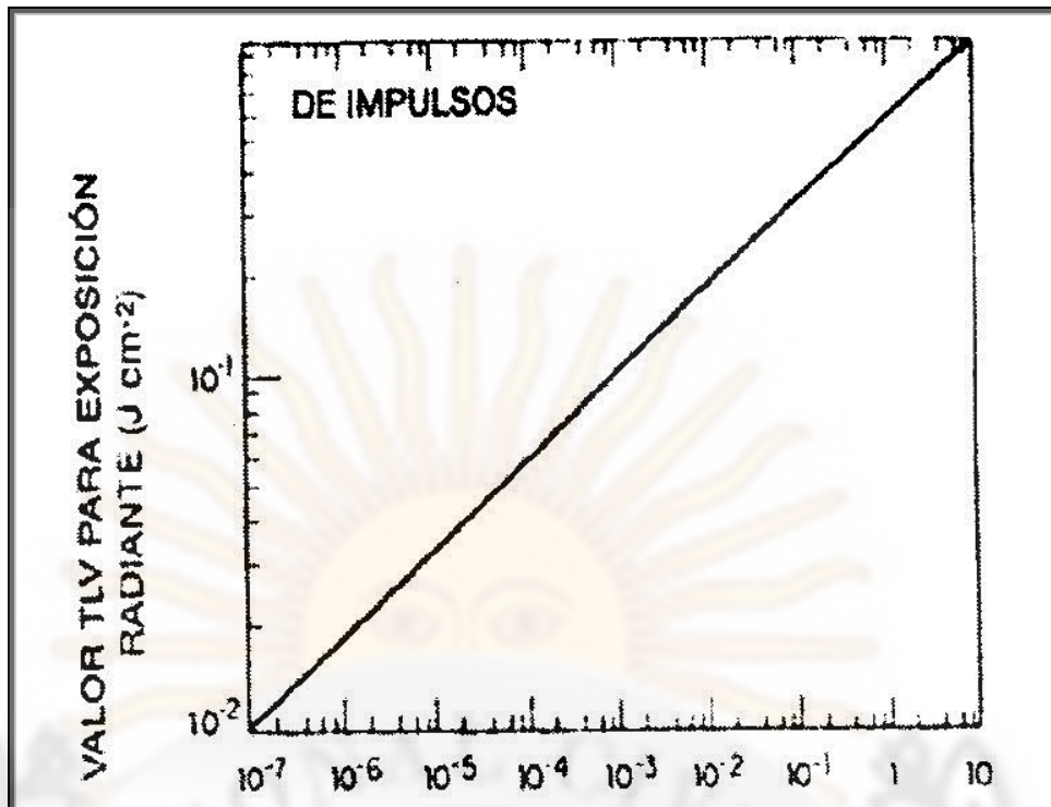
Figura 3a. Valor TLV para exposición de la piel y los ojos a láser para radiación infrarroja lejana. (Longitudes de onda superiores a 1,4 mm).
