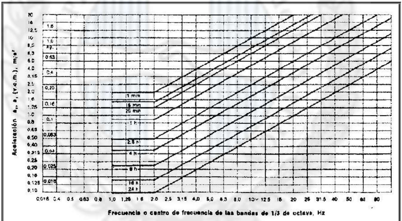
Figura 2. Límites de aceleración transversal ( a_x, a_y ) en función de la frecuencia y tiempo de exposición. Adaptado según ISO 26311
